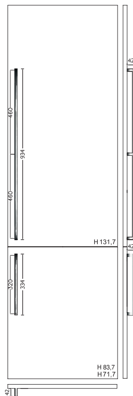
ANTA CESTELLO ESTRAIBILE PULL-OUT BASKET DRAWER DOOR
